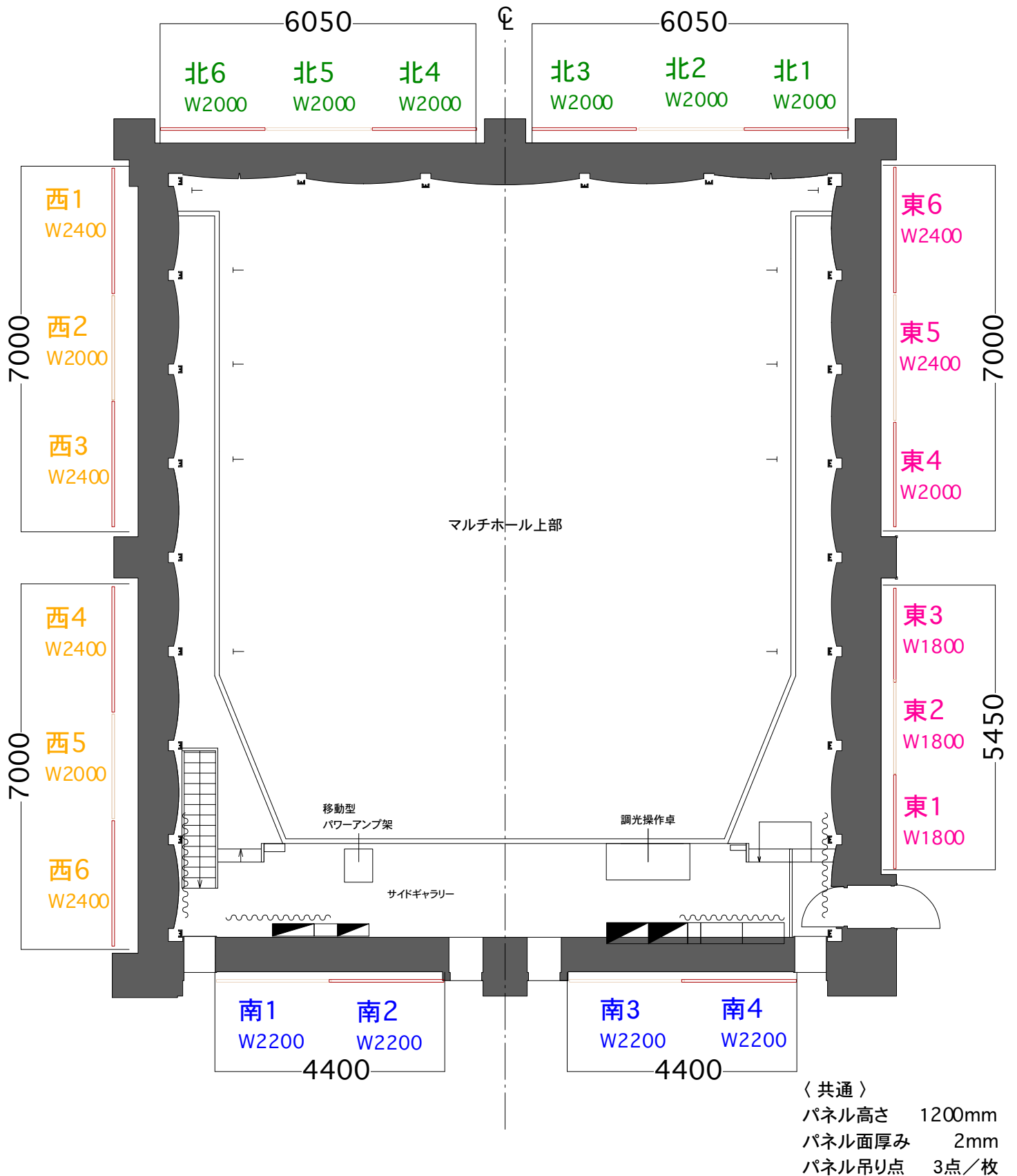
2階平面図
